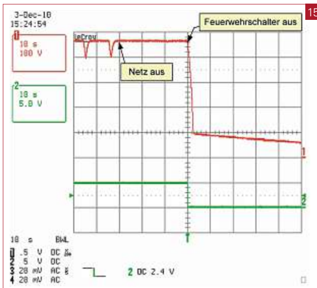
Fall 4: Verlauf der DC-Eingangsspannung am Solarmax 15MT bei simuliertem nächtlichem Schwachlichtbetrieb nach Öffnen des Feuerweherschalters (30 s nach Trennung vom Netz, PV-Generator mit U_{OC} = 500 V, I_{SC} = 60 mA, WR speist auch bei vorhandenem Netz nicht ein, maximale Spannung am Kondensator C_E wegen Belastung durch DC-ÜW etwas < U_{OC} ). CH1: DC-Spannung [100 V/Div]; CH2: Triggersignal [5 V/Div]; Zeitmassstab 10 s/Div. Bei diesem dreiphasigen Wechselrichter mit relativ kleinem C_E dauert es nur noch etwa 2 s, bis die Spannung an C_E auf 120 V gesunken ist.
