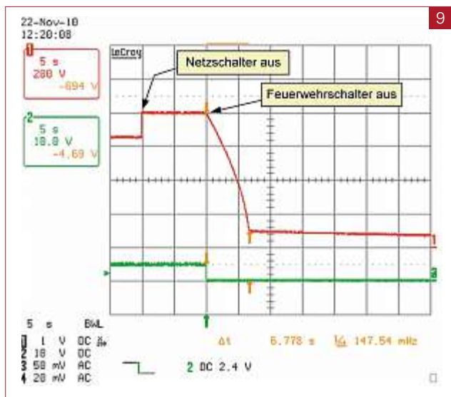
Fall 1: Netztrennung mit verzögerter (10 s) DC-Trennung durch Feuerwehrscharter am SolarMax 15MT bei einer Betriebsspannung von 650 V, U_{OC} = 810 V und I_{SC} = 25 A. CH1: DC-Spannung [200 V/Div]; CH2: Triggersignal [10 V/Div]; Zeitmassstab 5 s/Div. Bei diesem dreiphasigen Wechselrichter mit relativ kleinem C_E unterschreitet die DC-Spannung bereits 6,8 s nach dem Öffnen des Schalters den Grenzwert von 120 V.
