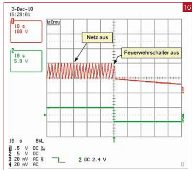
Fall 4: Verlauf der DC-Eingangsspannung am Solarmax 15MT bei simuliertem nächtlichem Schwachlichtbetrieb nach Öffnen des Feuerweherschalters (30 s nach Trennung vom Netz, PV-Generator mit U_{OC} = 500 V, aber I_{SC} = 20 mA, WR speist auch bei vorhandenem Netz nicht ein). Wegen des kleineren I_{SC} ist die maximale Spannung an C_E wegen Belastung durch DC-ÜW \ll U_{OC} (Belastungsversuche durch WR deutlich sichtbar). CH1: DC-Spannung [100 V/Div]; CH2: Triggersignal [5 V/Div]; Zeitmassstab 10 s/Div. Es dauert nur 1 s, bis die Spannung an C_E auf unter 120 V gesunken ist.
