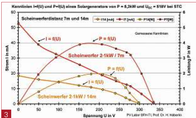
3 I-U- und P-U-Kennlinie eines Solargenerators aus 96 Modulen Siemens M55 (4 Stränge zu 24 Modulen in Serie) bei Bestrahlung mit 2 Halogenscheinwerfern von je 1 kW im Abstand von 7 m resp. 14 m.
