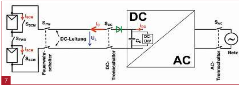
7 Prinzipschema einer PV-Anlage mit verschiedenen Möglichkeiten zur DC-seitigen Spannungsreduktion bei Bränden.
