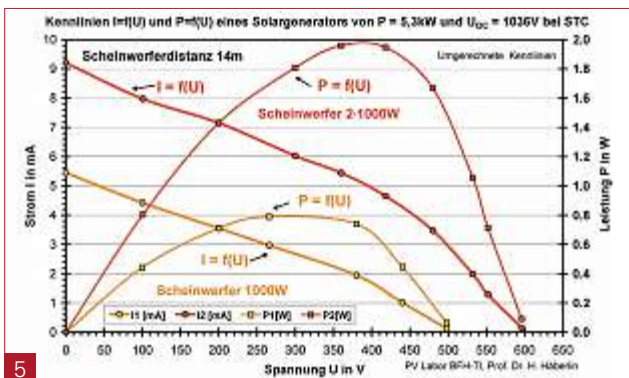
5 I-U- und P-U-Kennlinie eines Solargenerators aus 96 Modulen Siemens M55 (2 Stränge zu 48 Modulen in Serie) bei Bestrahlung im Abstand von 14 m mit einem oder zwei Halogenscheinwerfern von 1 kW (aus den Messungen von Abb. 4 für diesen Fall umgerechnete Kennlinien). Die Spannungen sind zwar doppelt so gross, die Ströme jedoch nur noch halb so gross.
