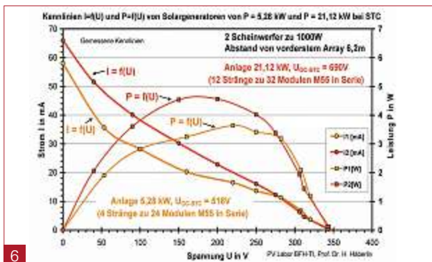
6 I-U- und P-U-Kennlinie eines PV-Generators von 21,1 kW aus 384 Modulen M55 (12 Stränge zu 32 Modulen in Serie) im Vergleich zum PV-Generator von Abb. 3 und 4 bei Bestrahlung im Abstand von 6,2 m mit zwei Halogenscheinwerfern von 1 kW. Da in jedem Strang ein Teil der Module ( \geq 8 ) viel weiter von den Scheinwerfern entfernt ist, ist die Bestrahlungsstärke sehr inhomogen. Nur I_{sc} steigt etwas, U_{oc} praktisch nicht!
