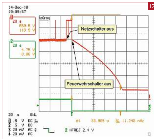
Fall 1: Netztrennung mit verzögerter (10 s) DC-Trennung durch Feuerwehrscharter am SMC 8000TL bei einer Betriebsspannung von 525 V, U_{OC} = 656 V und I_{SC} = 16 A. CH1: DC-Spannung [100 V/Div]; CH2: Triggersignal [5 V/Div]; Zeitmassstab 20 s/Div. Bei diesem grossen einphasigen Wechselrichter wird ein grosser Eingangskondensator C_E benötigt. Deshalb dauert es etwa 89 s, bis die Spannung an C_E auf 120 V gesunken ist.
