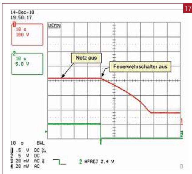
17 Fall 4: Verlauf der DC-Eingangsspannung am SMC 8000TL bei simuliertem nächtlichem Schwachlichtbetrieb nach Öffnen des Feuerweherschalters (30 s nach Trennung vom Netz, PV-Generator mit U_{oc} = 328 V, I_{sc} = 60 mA, WR speist auch bei vorhandenem Netz nicht ein). CH1: DC-Spannung [100 V/Div]; CH2: Triggersignal [5 V/Div]; Zeitmassstab 10 s/Div. Bei diesem grossen einphasigen Wechselrichter mit einem grossen C_E dauert es auch hier noch etwa 34 s, bis die Spannung an C_E auf unter 120 V gesunken ist.
