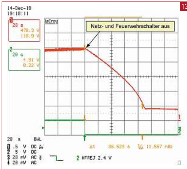
Fall 2: Gleichzeitige Trennung von Netzschalter und Feuerweherschalter am SMC 8000TL bei einer Betriebsspannung von 525 V, U_{OC} = 656 V und I_{SC} = 16 A. CH1: DC-Spannung [100 V/Div]; CH2: Triggersignal [5 V/Div]; Zeitmassstab 20 s/Div. Es dauert etwa 86 s, bis die Spannung an C_E auf 120 V gesunken ist.
