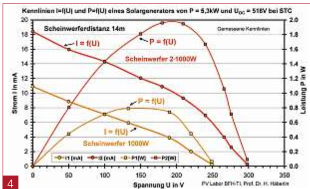
4 I-U- und P-U-Kennlinie eines Solargenerators aus 96 Modulen Siemens M55 (4 Stränge zu 24 Modulen in Serie) bei Bestrahlung im Abstand von 14 m mit einem oder zwei Halogenscheinwerfern von 1 kW.
