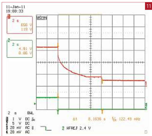
Fall 3: Trennung des Feuerwehrscharters bei noch laufendem Netz am SolarMax 15MT bei einer Betriebsspannung von 650 V, U_{OC} = 810 V und I_{SC} = 25 A. CH1: DC-Spannung [200 V/Div]; CH2: Triggersignal [5 V/Div]; Zeitmassstab 2 s/Div. Es dauert etwa 8,2 s, bis die Spannung an C_E auf 120 V gesunken ist.
