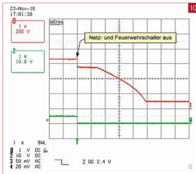
Fall 2: Gleichzeitige Trennung von Netz- und Feuerwehrscharter am SolarMax 15MT bei einer Betriebsspannung von 650 V, U_{OC} = 810 V und I_{SC} = 25 A. CH1: DC-Spannung [200 V/Div]; CH2: Triggersignal [10 V/Div]; Zeitmassstab 1 s/Div. Es dauert nur noch etwa 4,8 s, bis die Spannung an C_E auf 120 V gesunken ist.
