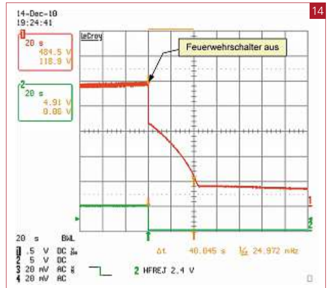
Fall 3: Trennung des Feuerweherschalters bei noch laufendem Netz am SMC 8000TL bei einer Betriebsspannung von 525 V, U_{OC} = 656 V und I_{SC} = 16 A. CH1: DC-Spannung [100 V/Div]; CH2: Triggersignal [5 V/Div]; Zeitmassstab 20 s/Div. Es dauert nur noch etwa 40 s, bis die Spannung an C_E auf 120 V gesunken ist. Das Netz würde hier am besten kurz nach dem Feuerweherschalter abgeschaltet, dann entlädt der zunächst noch laufende Wechselrichter C_E auf die minimal mögliche Betriebsspannung.
