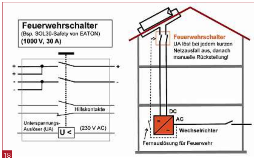
18 Feuerweherschalter beim PV-Generator.
